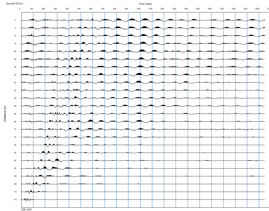
Sismograma correspondiente a datos de adquisición MASW-01
