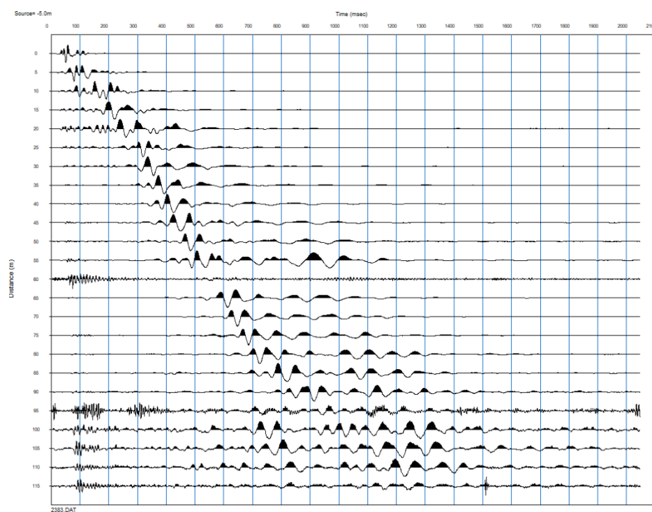
Sismograma correspondiente a datos de adquisición MASW-02
