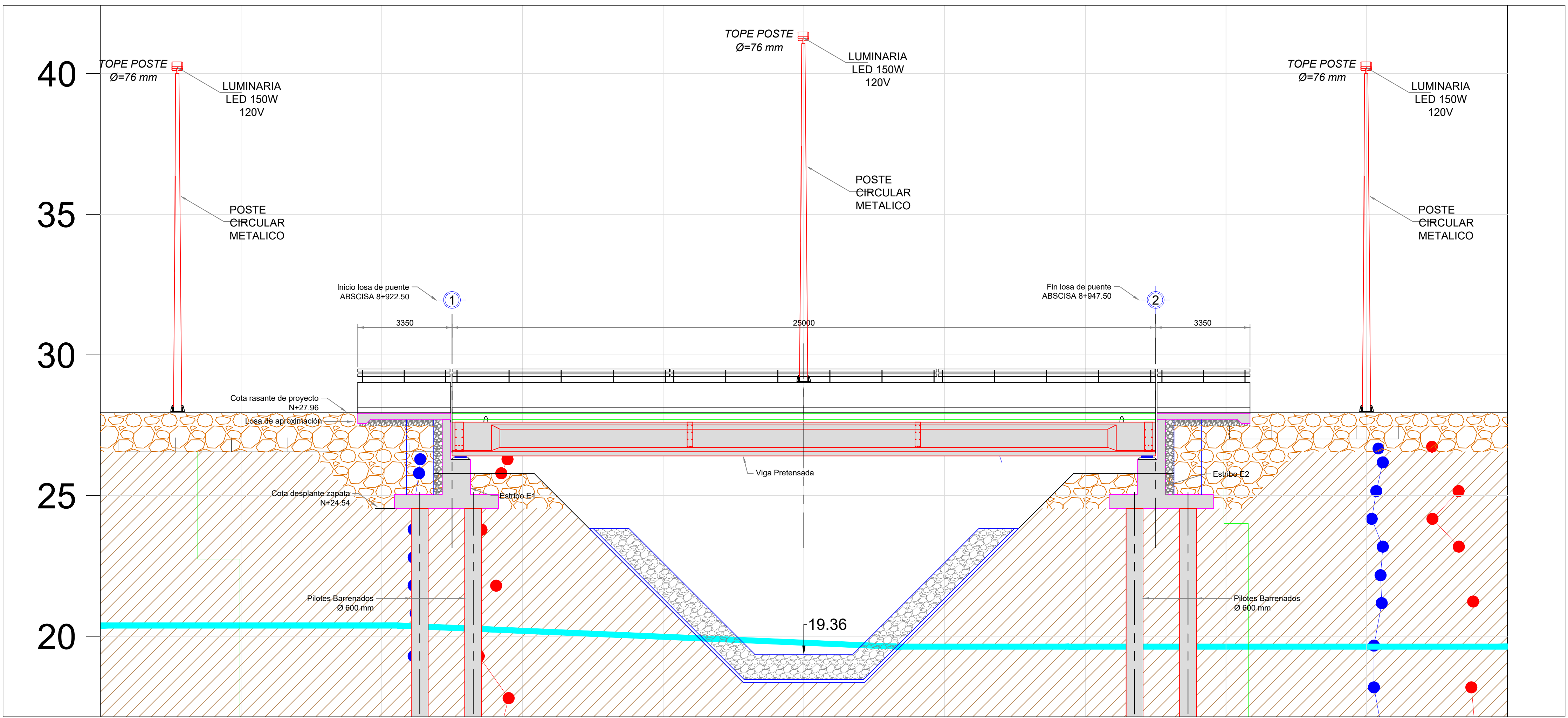
ELEVACION
